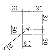
PEÇA C CHAPA # 3/8" QUANTIDADE : 06 PÇS
