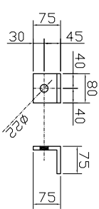
PEÇA B CANTONEIRA L 3"x3" x 3/8" QUANTIDADE : 24 PÇS
